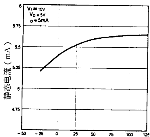
静态电流
